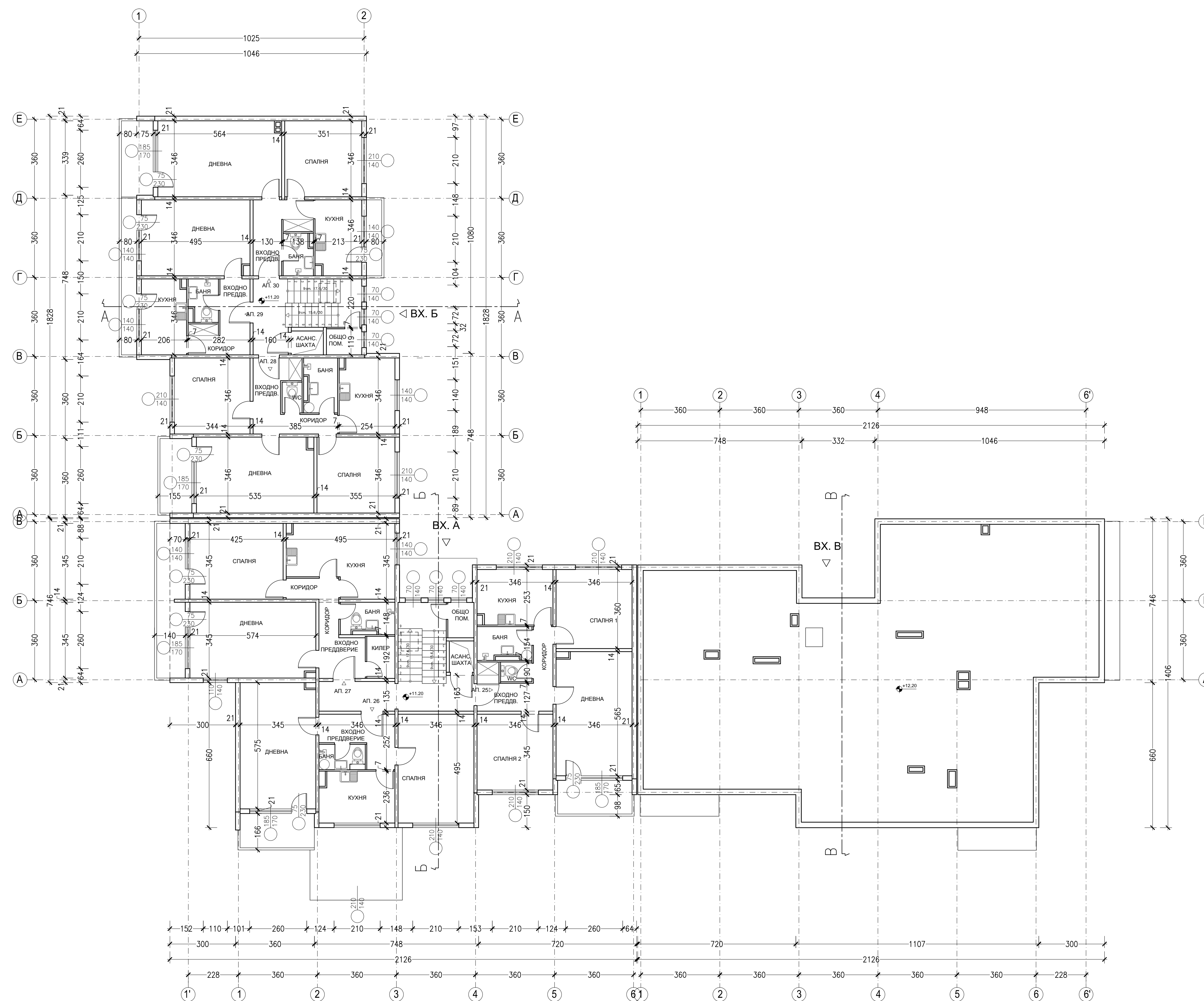
ПЛАН КОТА +11.20
