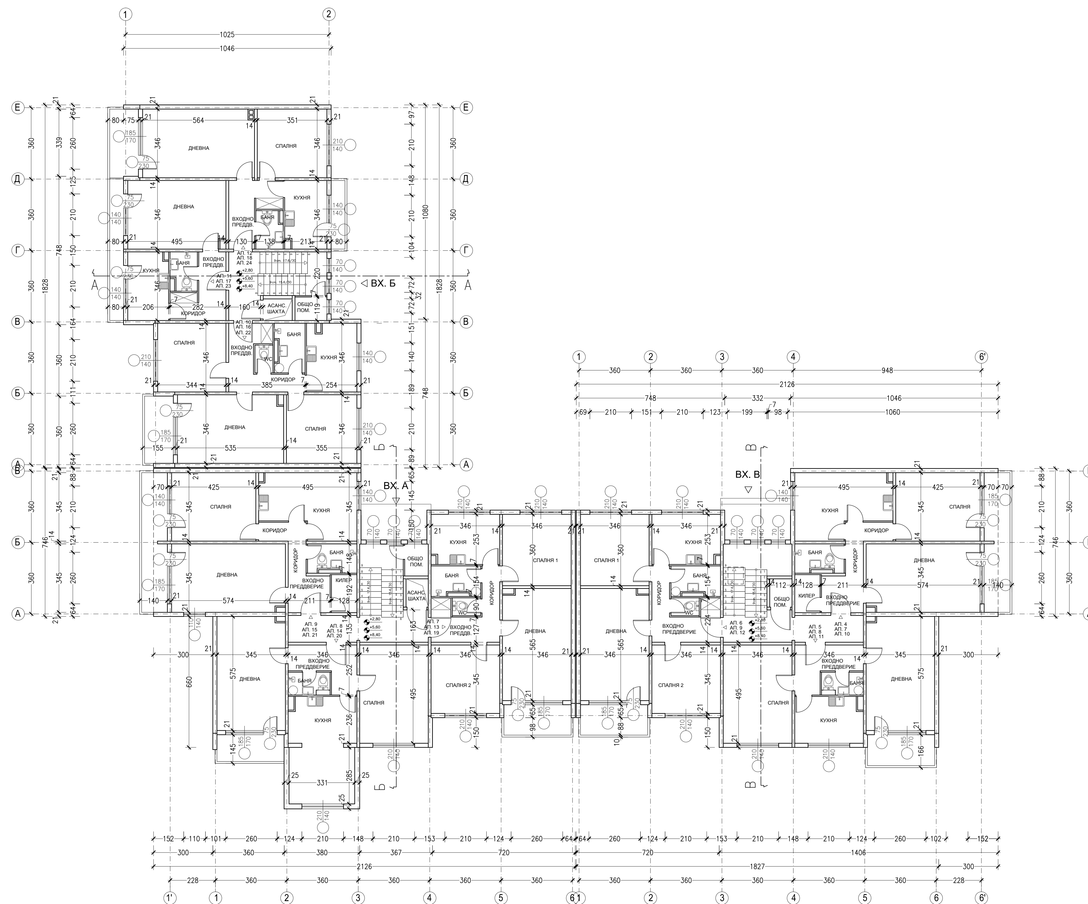
ПЛАН ТИПОВ ЕТАЖ КОТА +2.80 +5.60 +8.40
