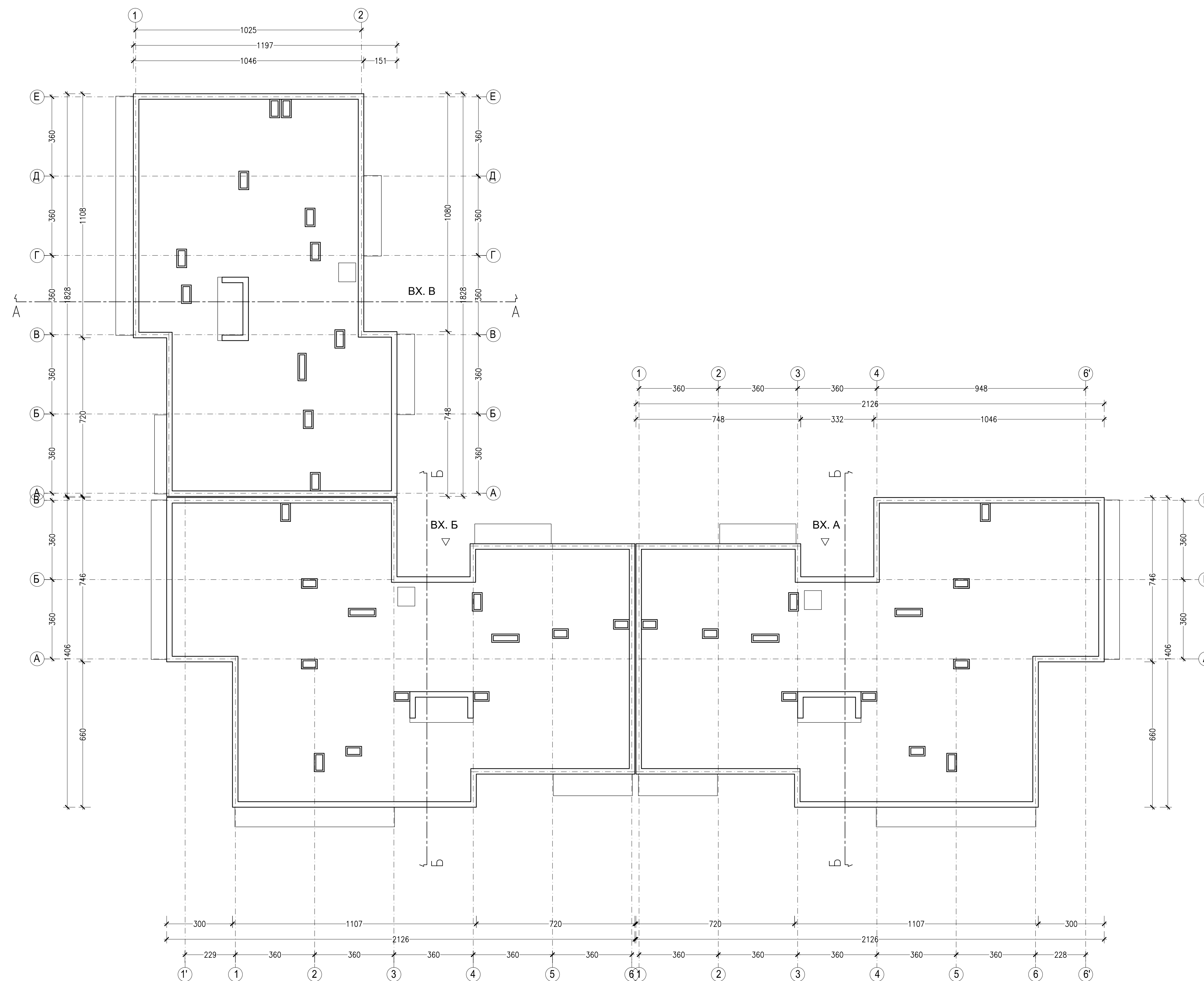
ПЛАН КОТА +11.20
