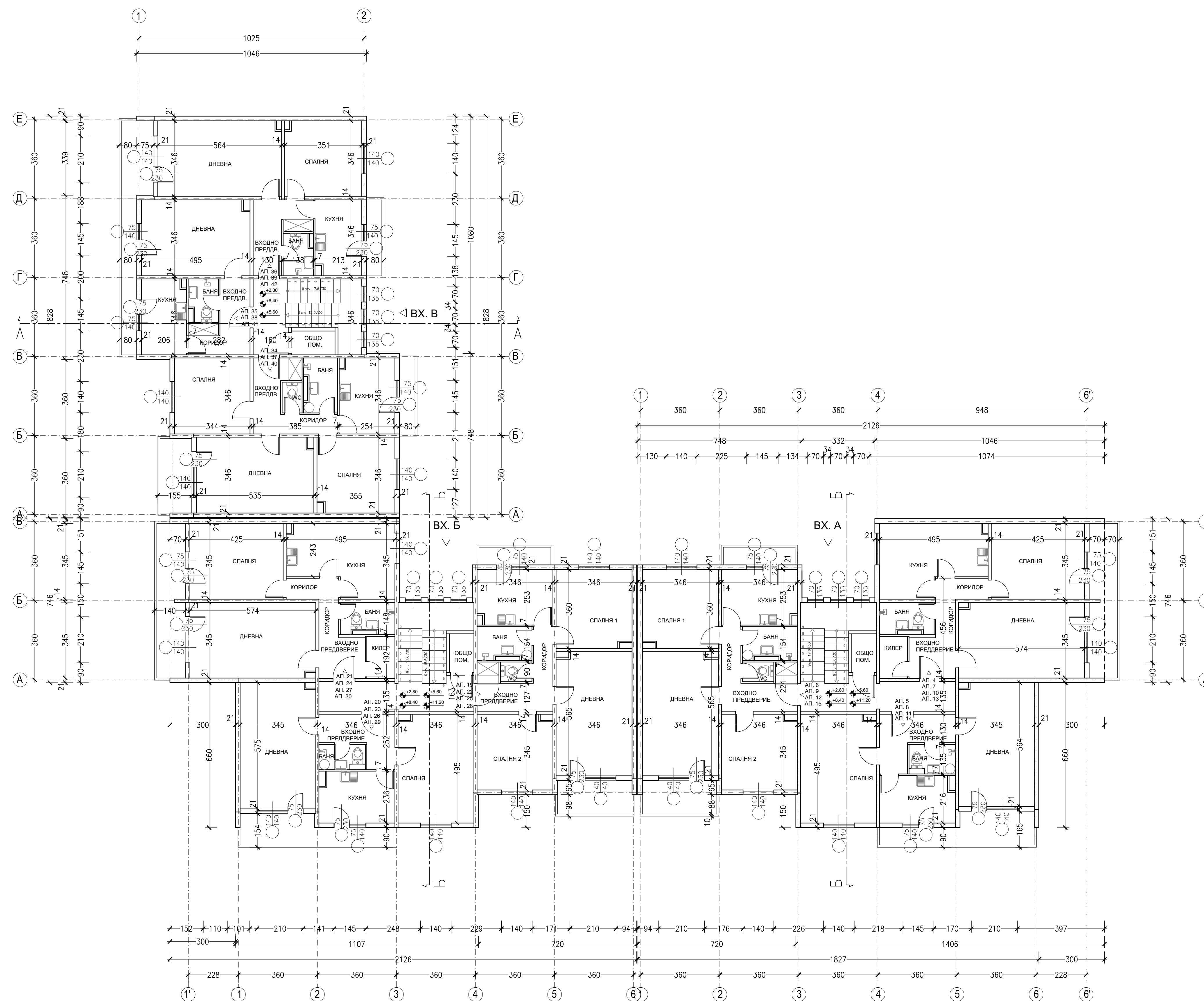
ПЛАН ТИПОВ ЕТАЖ КОТА +2.80 +5.60 +8.40 +11.20
