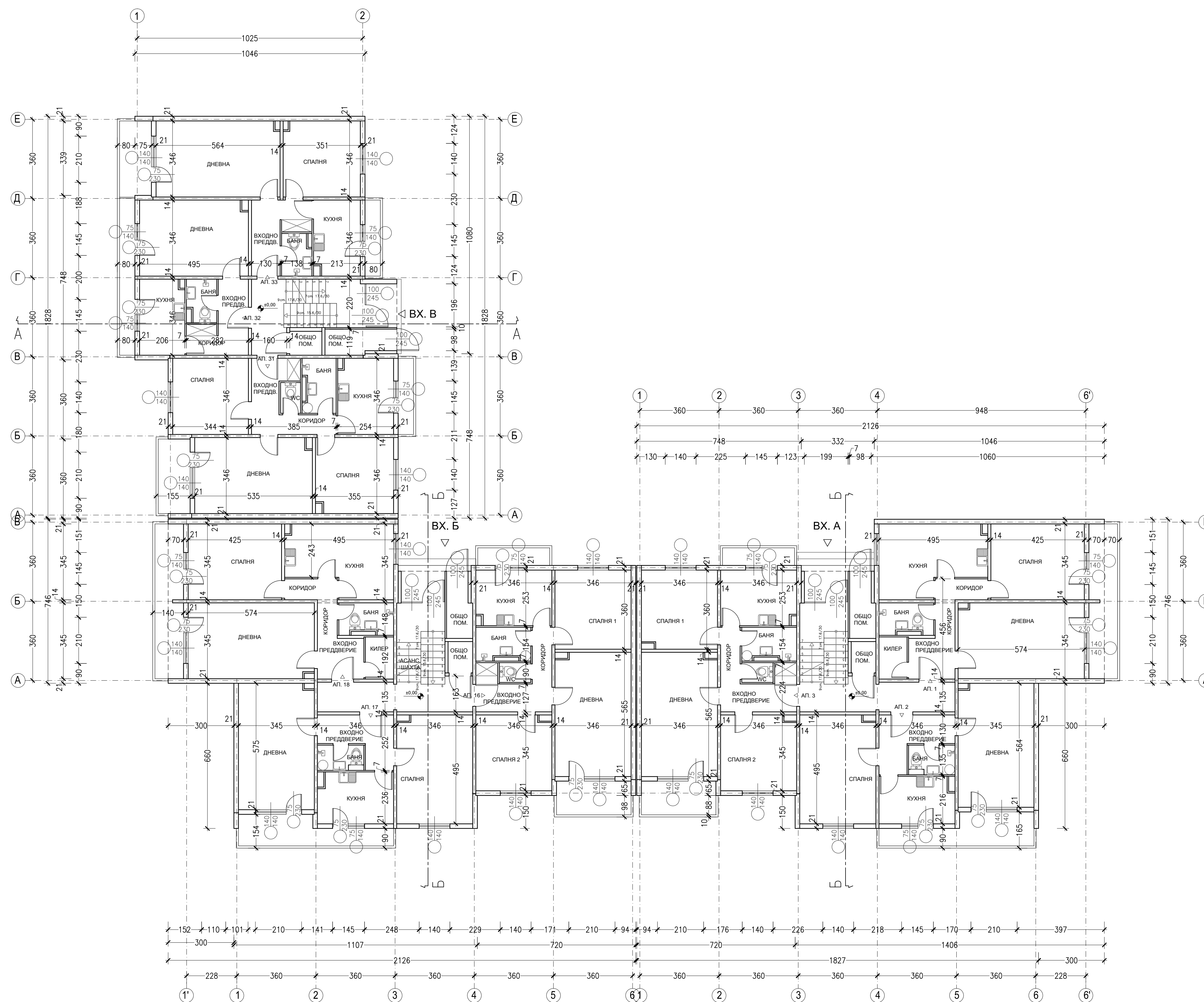
ПЛАН ПЪРВИ ЕТАЖ КОТА ±0.00
