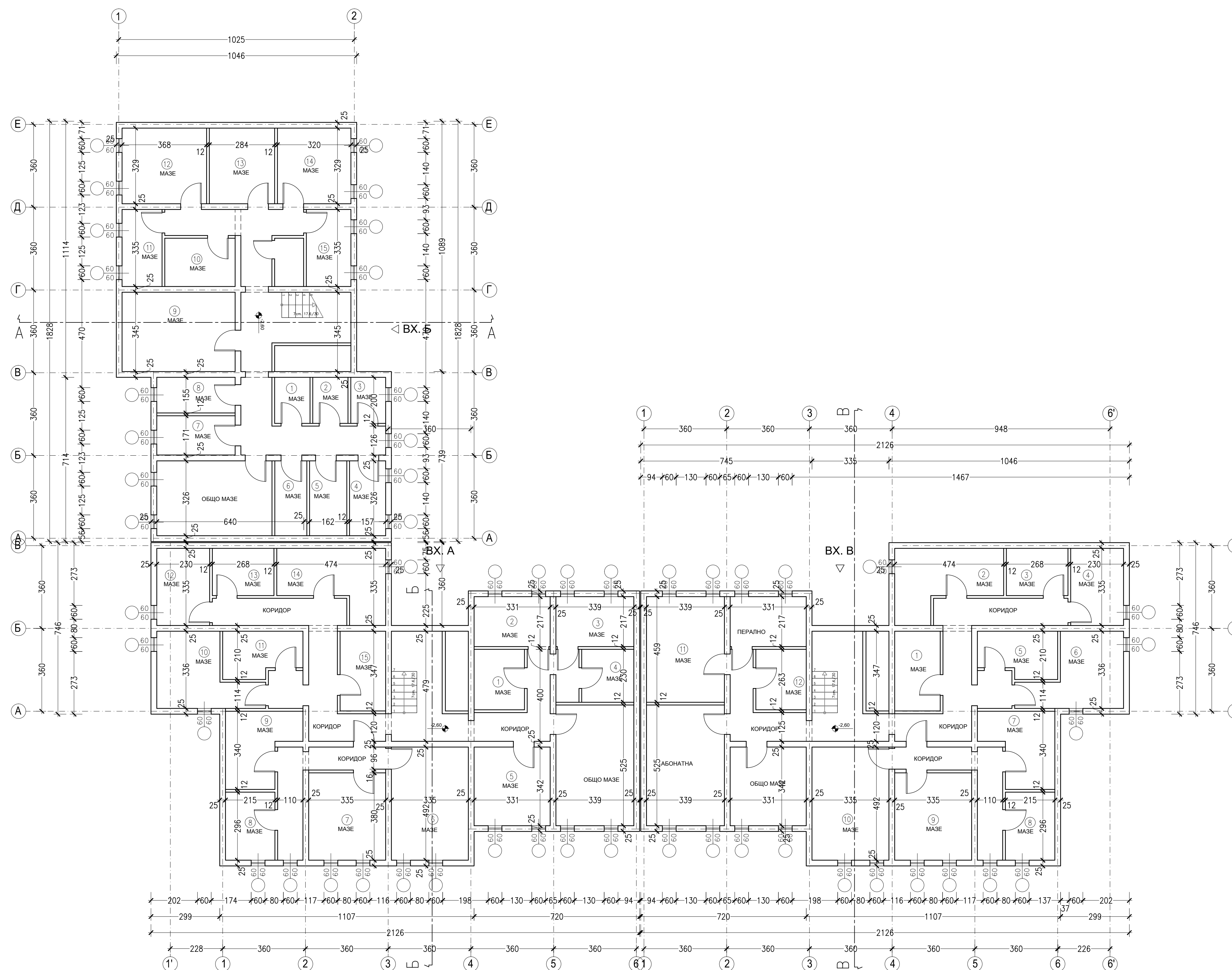
ПЛАН СУТЕРЕН КОТА -2.60
